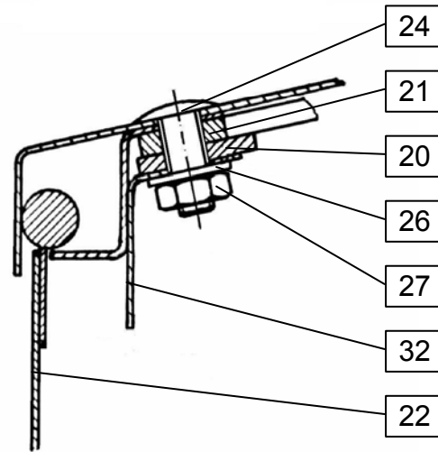
PREREZ B-B
