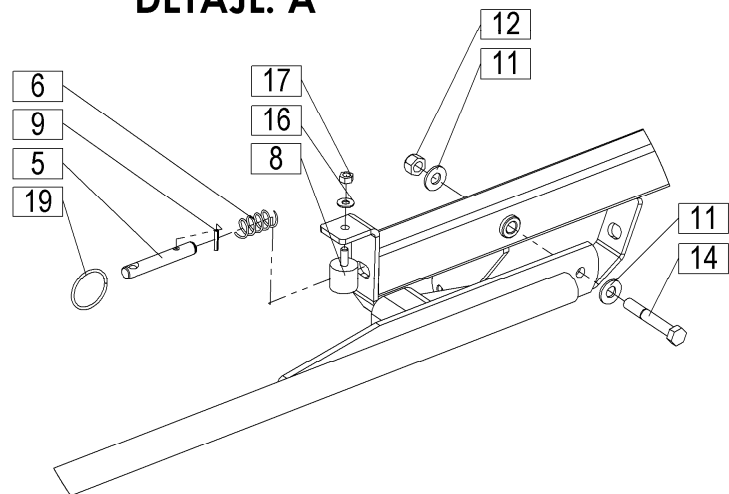
DETAJL: A
