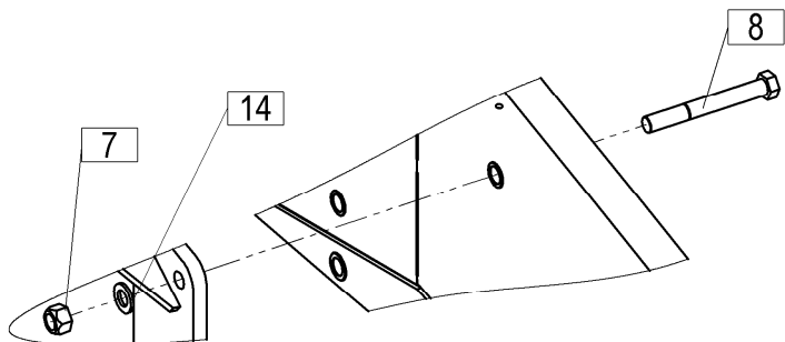
DETAJL: A
