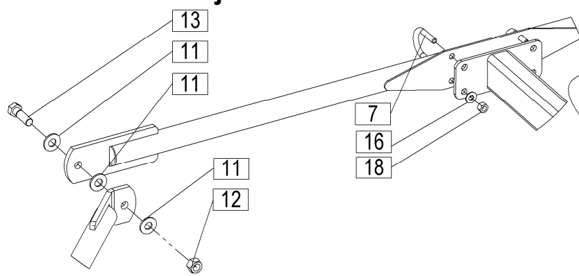
Detajl: C
