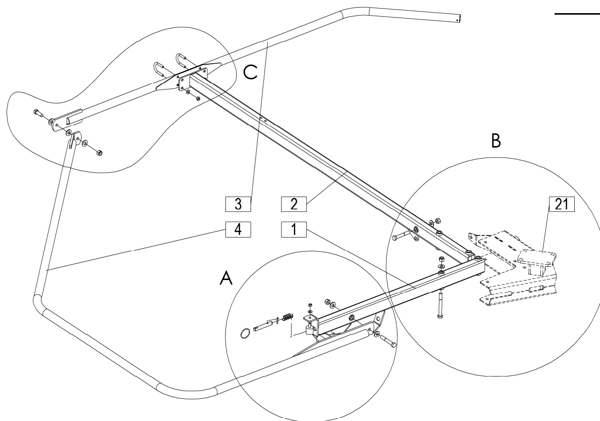
DETAJL: C
