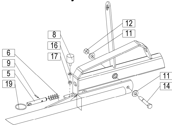
Detajl: A
