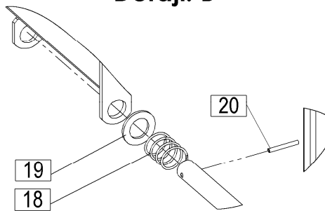
Detajl: B
