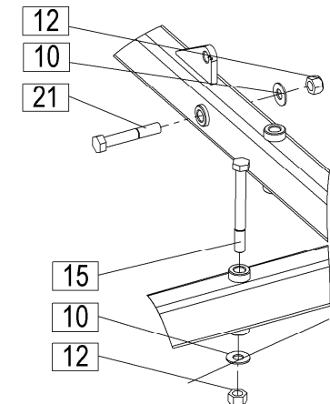
Detajl: B
