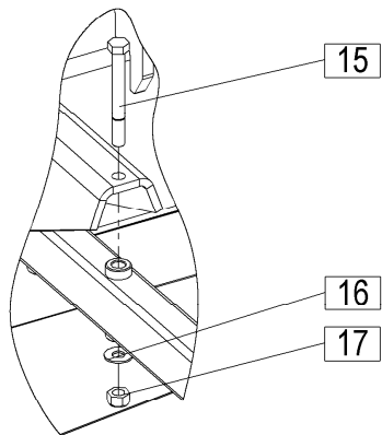
Detajl: A
